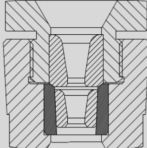
Typ BT mit HM-Einsatz
