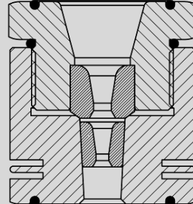
Typ BS mit O-Ring Dichtungen
