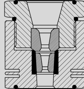
Typ BS mit O-Ring Dichtungen & HM-Einsatz
